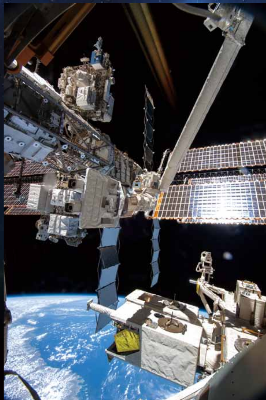
「きぼう」船内実験室(PM)の窓から見た 小型衛星放出機構(J-SSOD)©JAXA / NASA
